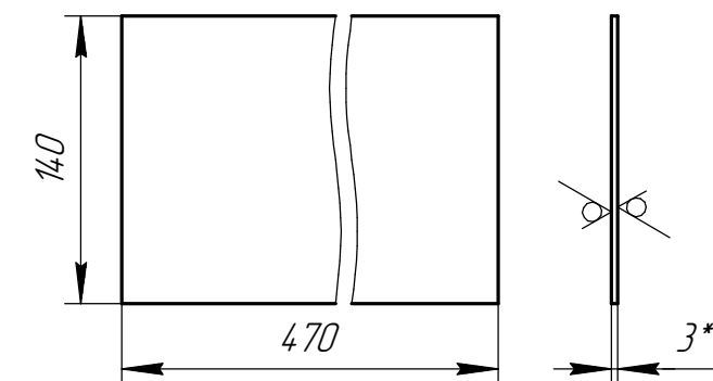
Дет. поз. 1
